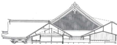
現状 中門梁間断面図
